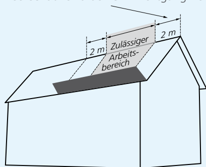
Dachschutzblende
