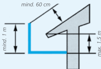
Dachfanggerüst
