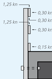
Lastanforderungen für die Bemessung von Wehren
